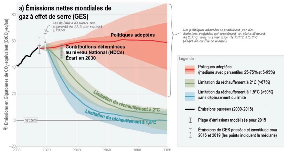
Figure 17 – Trajectoires et objectifs climatiques : des efforts supplémentaires et immédiats sont nécessaires Source : AR6 GIEC (traduit par Sydney Thomas pour BonPote)
